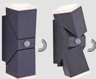
4609735. Anthrazit, Ausschaltverzögerung (6s-10 min), Reichweite (8 m), Dämmerungssensor (5 lux-2000 lux), 2 x 5 W, 3000 K, 700 lm, H 105-125, L 220, B 140, A 165-220 € 187,90
