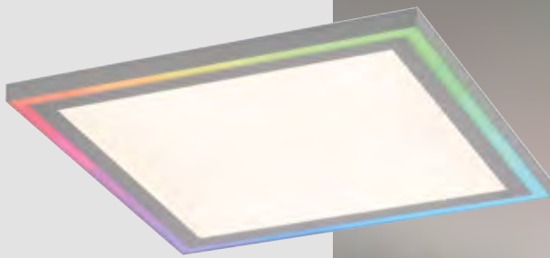
2629339. Weiß, innen CCT, außen RGB-Rainbow, Funkfernbedienung, 16 W LED, 2700-6000 K, 2300 lm, 5 W LED RGB, 2700-6000 K, L 400, B 400, H 52 € 198,90
